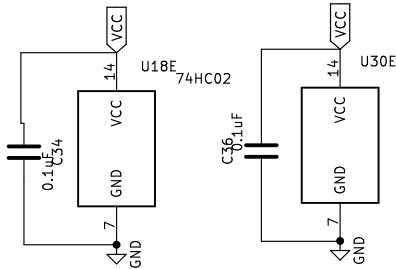
74HC02
